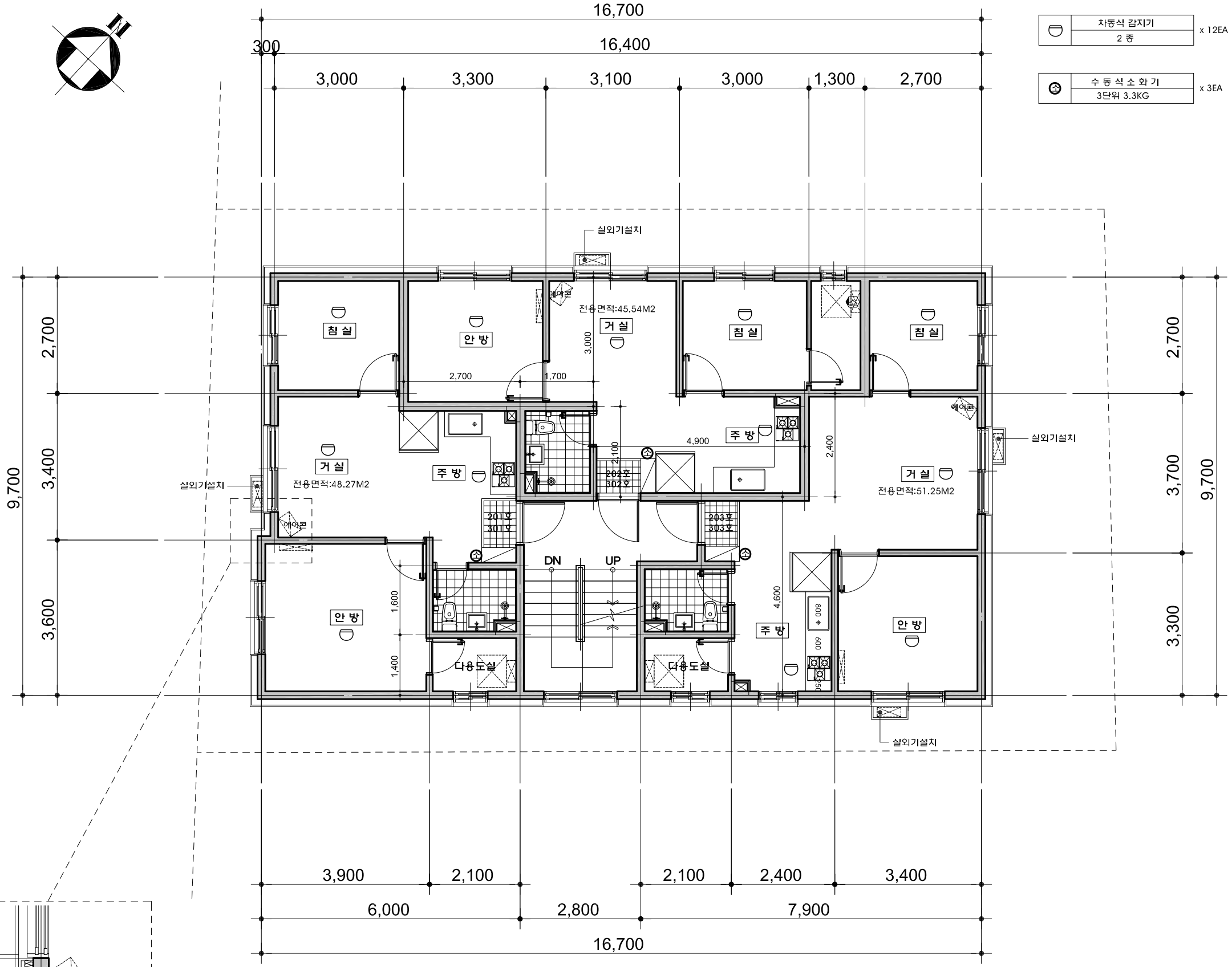
2~3 층 평 면 도 SCALE:1/100
