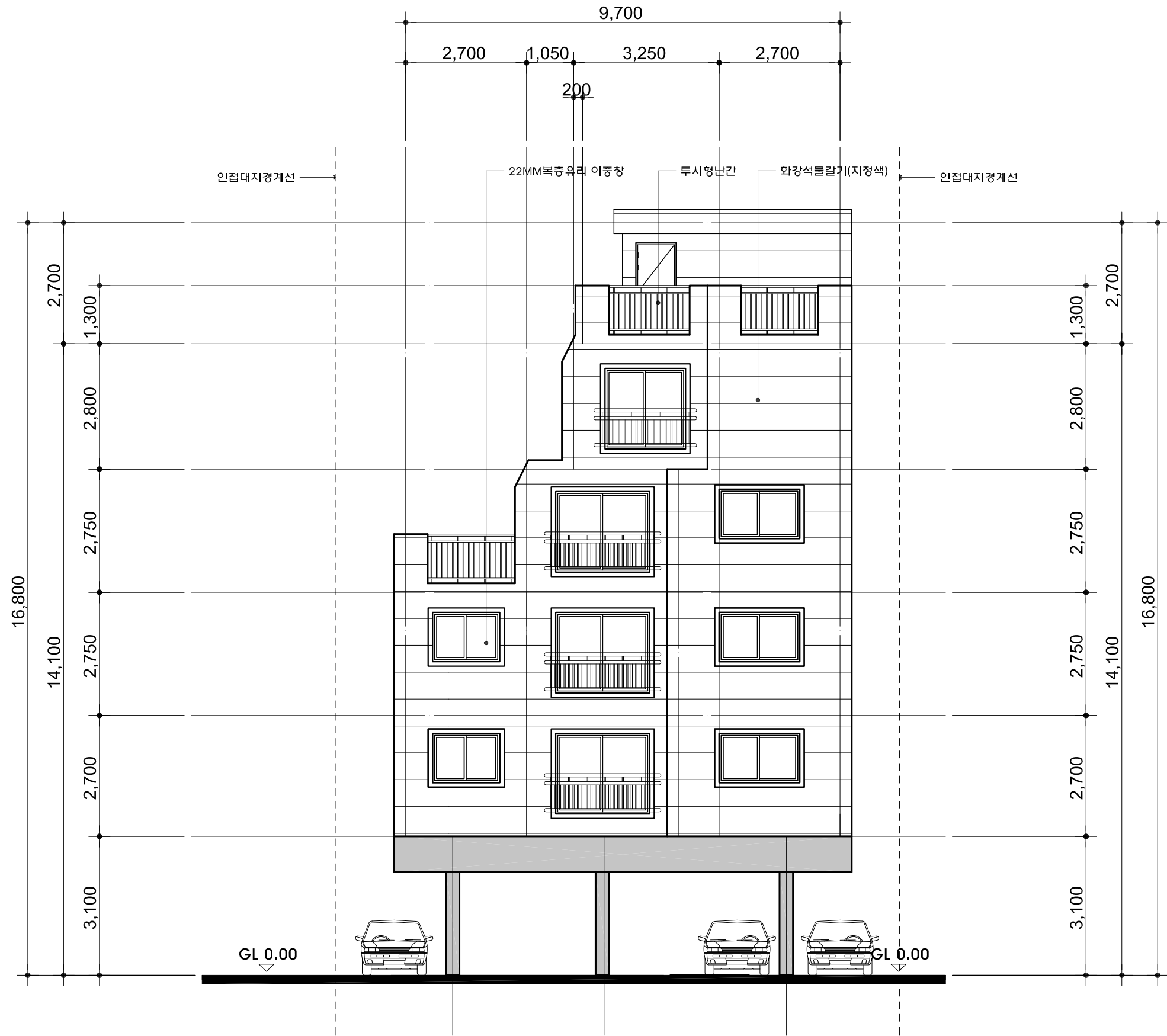
정 면 도 (동 측 면 도) SCALE:1/100
