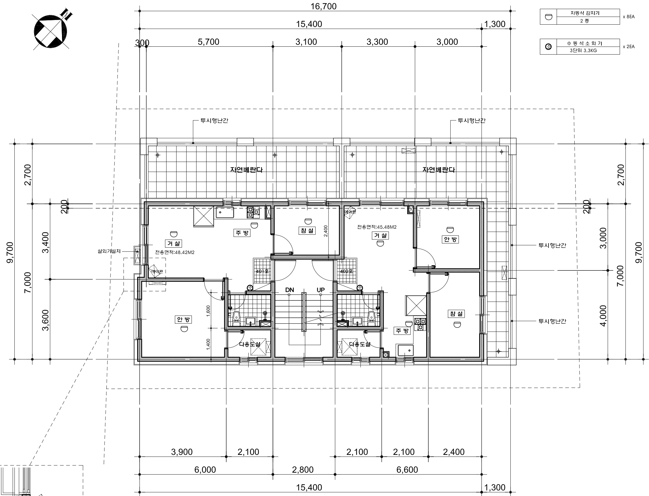
4 층 평 면 도 SCALE:1/100
