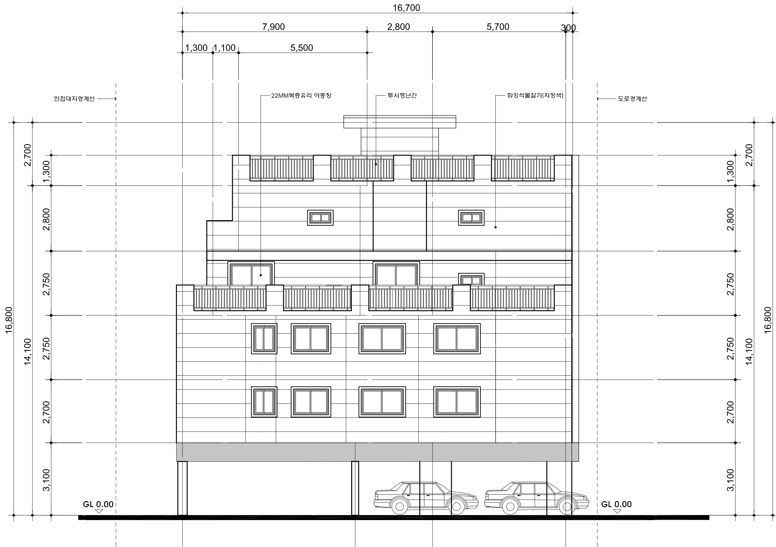
좌 측 면 도 (서 측 면 도) SCALE:1/100
