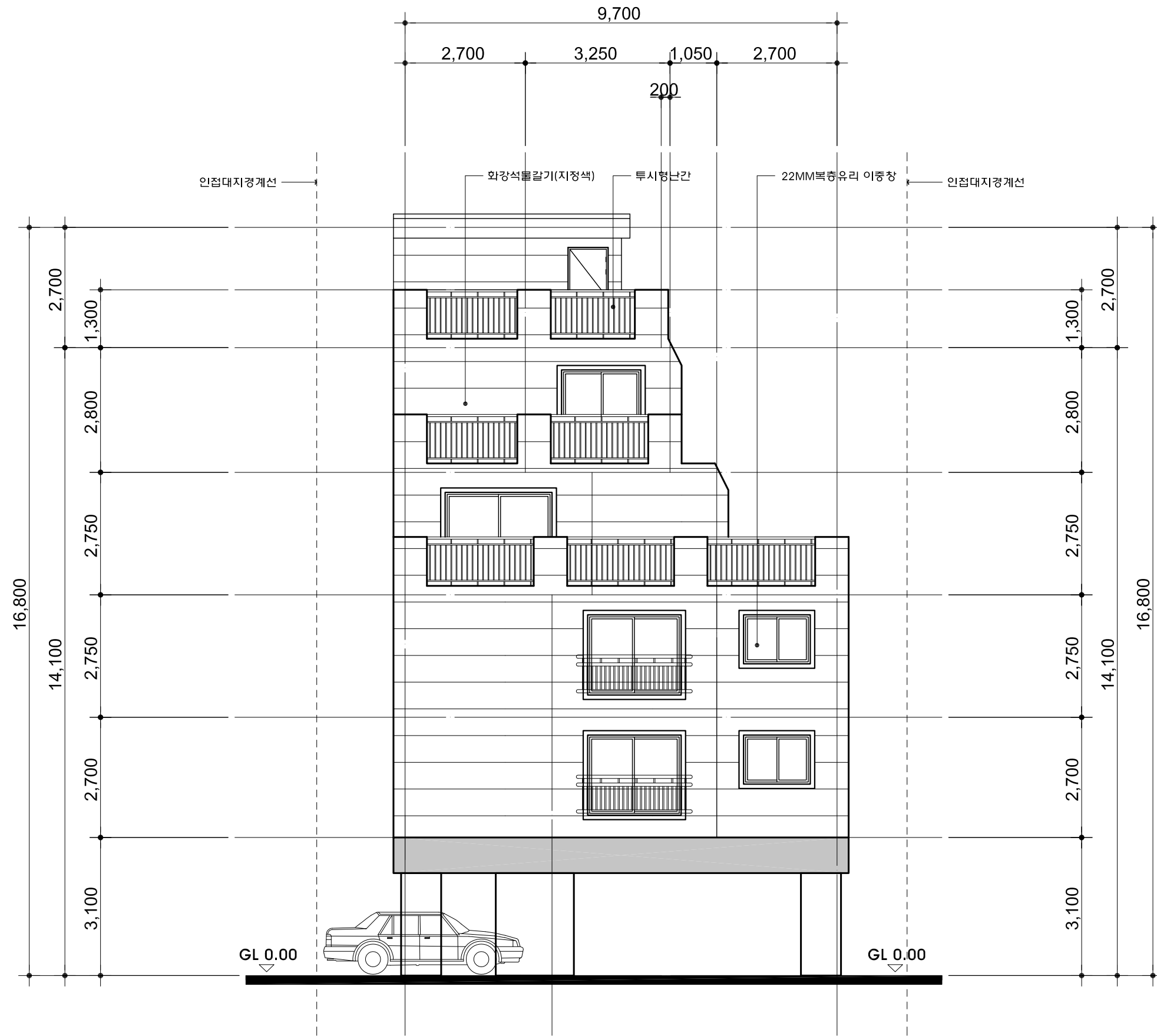
배 면 도 (서 측 면 도) SCALE:1/100
