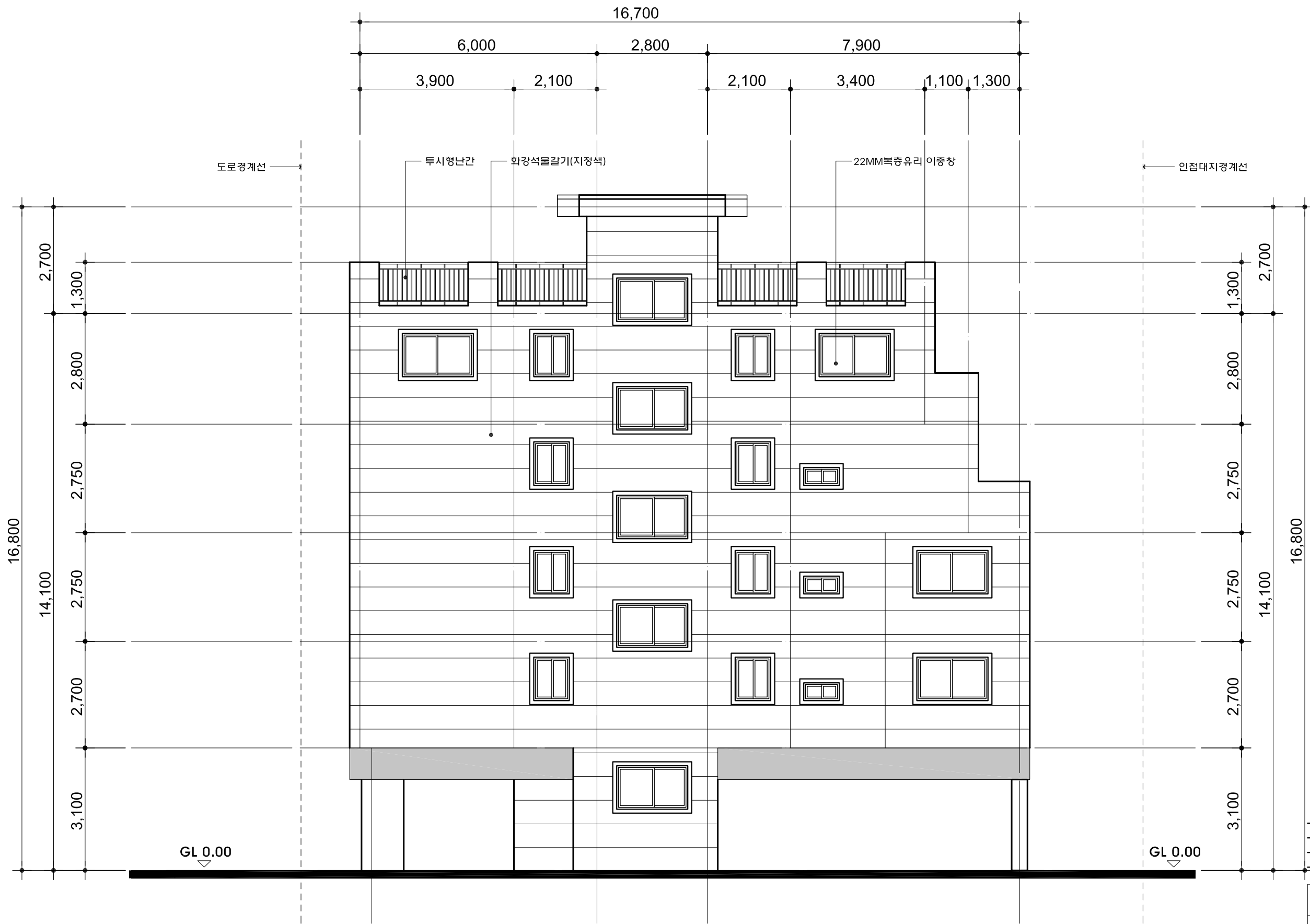
우 측 면 도 (북 측 면 도) SCALE:1/100
